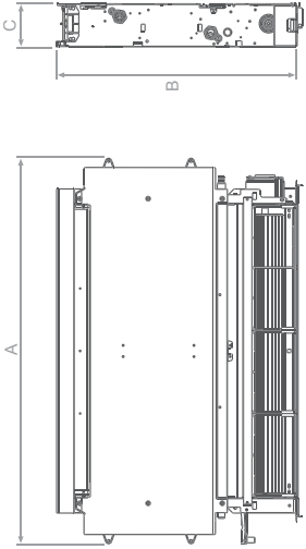
VERSIONE SLI 2 tubi da incasso (senza piastra radiante)
